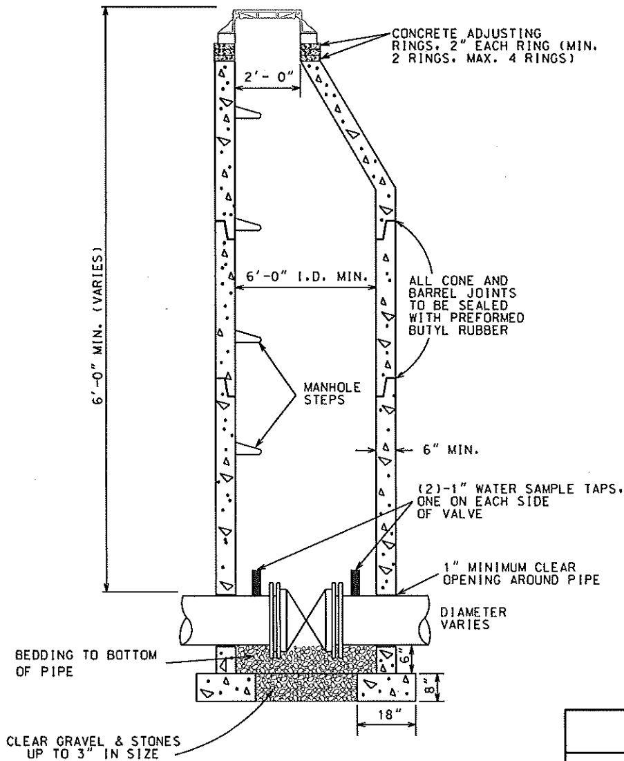
SECTION "A" N.T.S.
