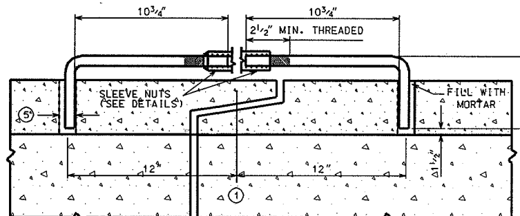
LONGITUDINAL SECTION
