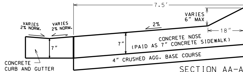
SECTION AA-AA
