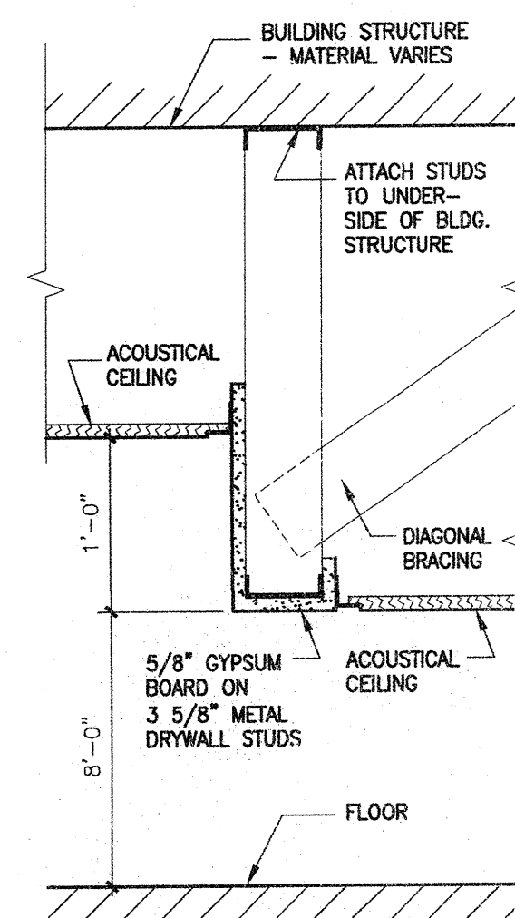
4 A301 SOFFIT SECTION SCALE: 1 1/2" = 1'-0"
