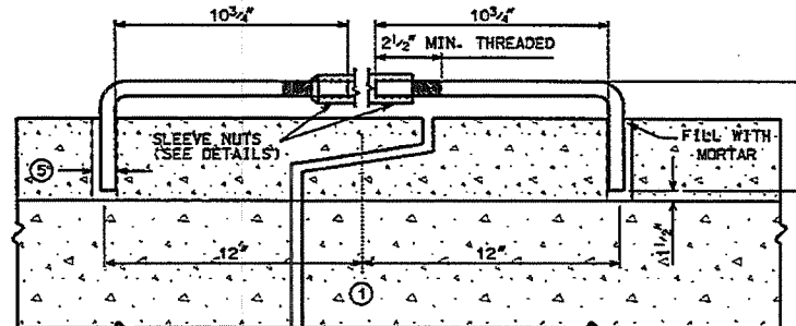
LONGITUDINAL SECTION
