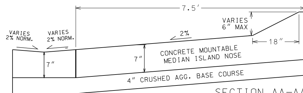
SECTION AA-AA
