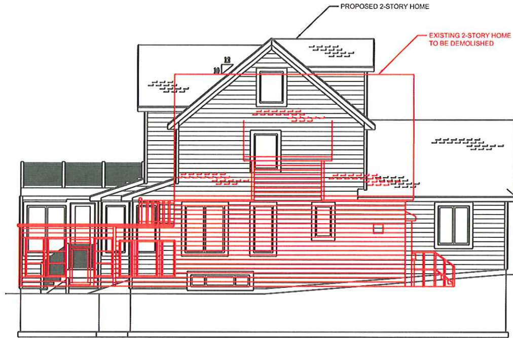
LEFT ELEVATION SCALE: 1/8"=1'
