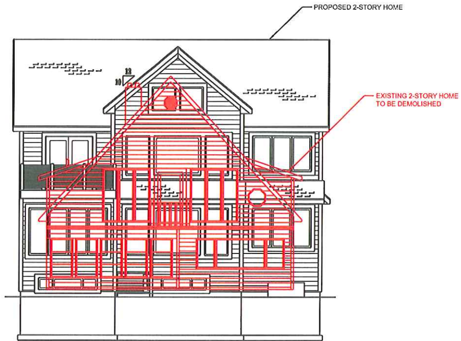
REAR ELEVATION SCALE: 1/8"=1'
