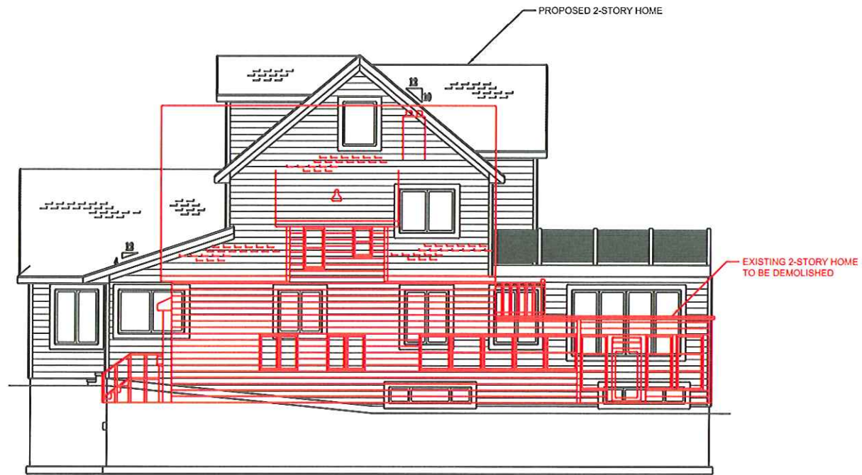
RIGHT ELEVATION SCALE: 1/8"=1'
